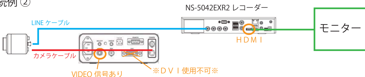
接続例②
